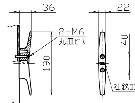
クリート詳細図
